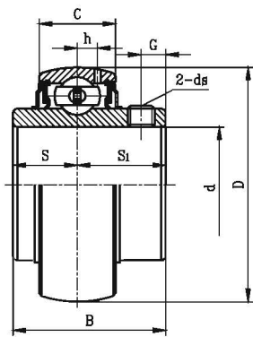
UC2 Setescrew type
